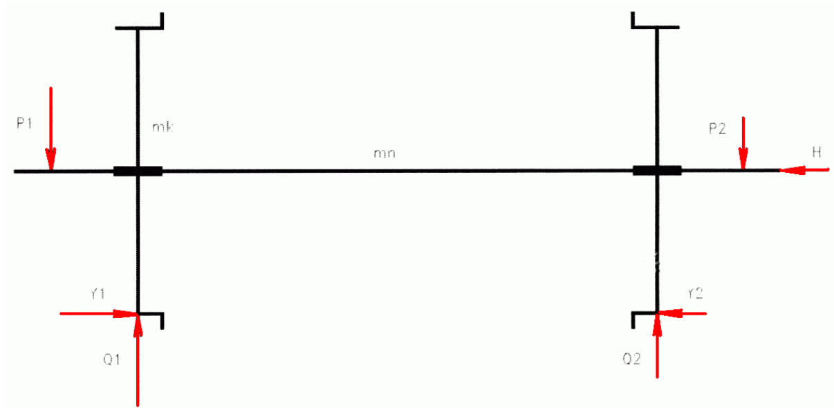
Výpočtový model nápravy železničního vagonu dle normy EN 13103 : 2001
